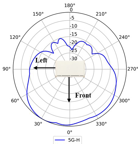
5GHz (Horizontal)
