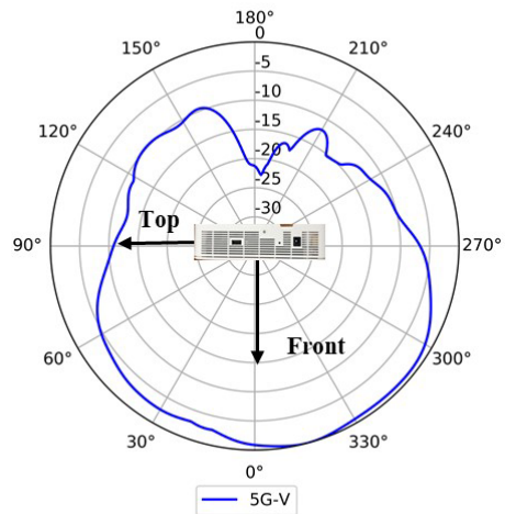
5GHz (Vertical)
